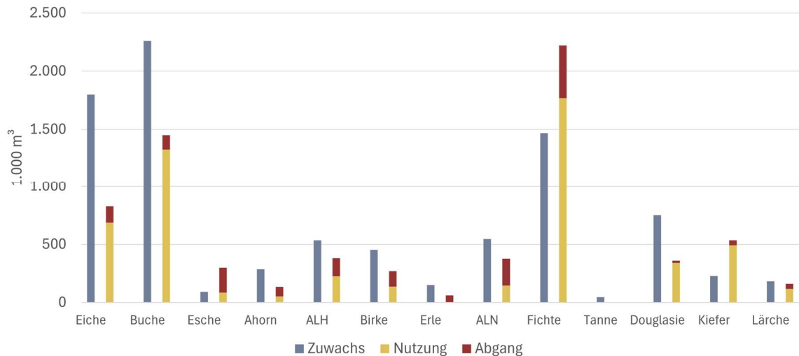
Abbildung 15: Zuwachs, Nutzung und Abgang über Baumartengruppen zwischen BWI III und BWI IV in 1.000 m 3
